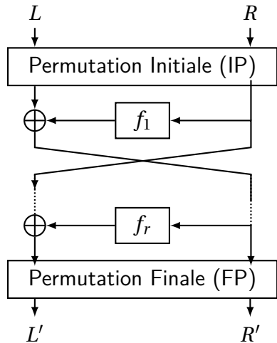
Schéma de Feistel (ex : DES)
