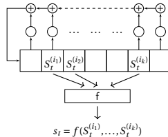
LFSR Filtrés
