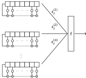
LFSR Combinés
